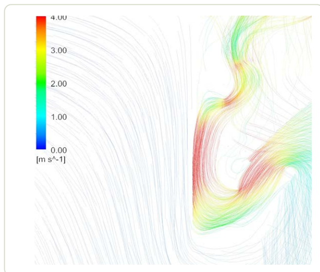
CFD simulace proudění vzduchu · rychlost 0–4 m/s.
